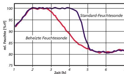
Nach einer Betauungsphase mit 100 % relativer Feuchte misst die beheizte Sonde sofort die korrekte Feuchte, während eine nicht beheizte Sonde einige Zeit benötigt, um sich von der Betauung zu erholen.
