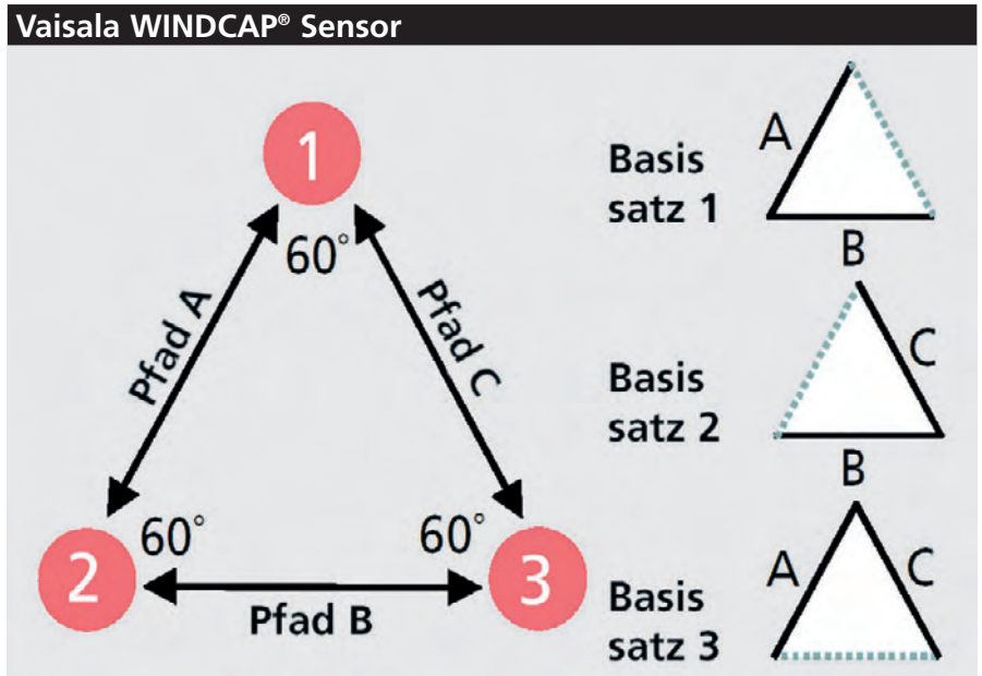
Die Anordnung der Schallköpfe als gleichseitiges Dreieck stellt drei Gruppen von Basisvektoren zur Verfügung und ermöglicht in dieser Kombination bi-direktionale Messungen entlang der Schallpfade A, B und C. Die Messergebnisse dienen zur Bestimmung der Windgeschwindigkeitskomponenten parallel zu den Pfaden.
