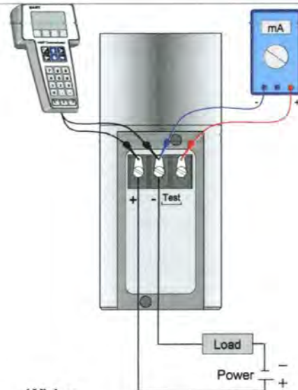
Wiring
