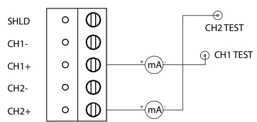
2) Analogausgangstest
