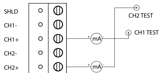
2) Teste da saída analógica
