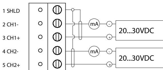
1) Diagrama da fiação
