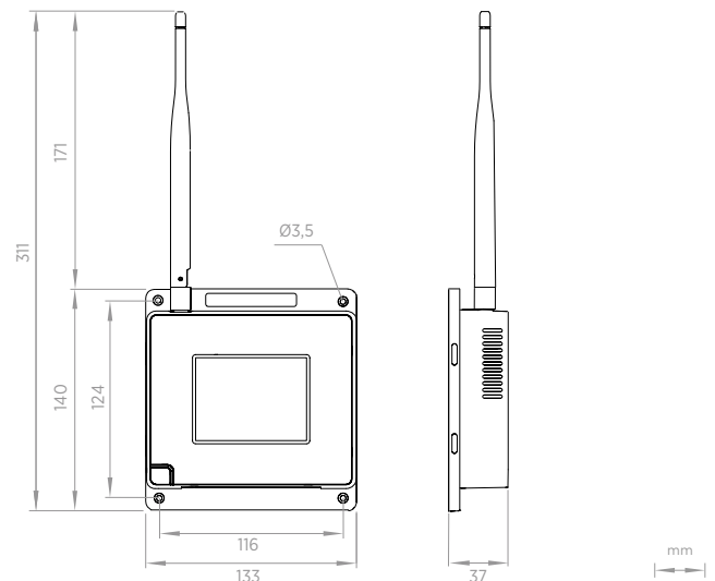
CA10 Abmessungen
