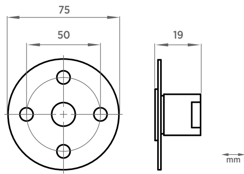
Abmessungen Montageflansch 210696
