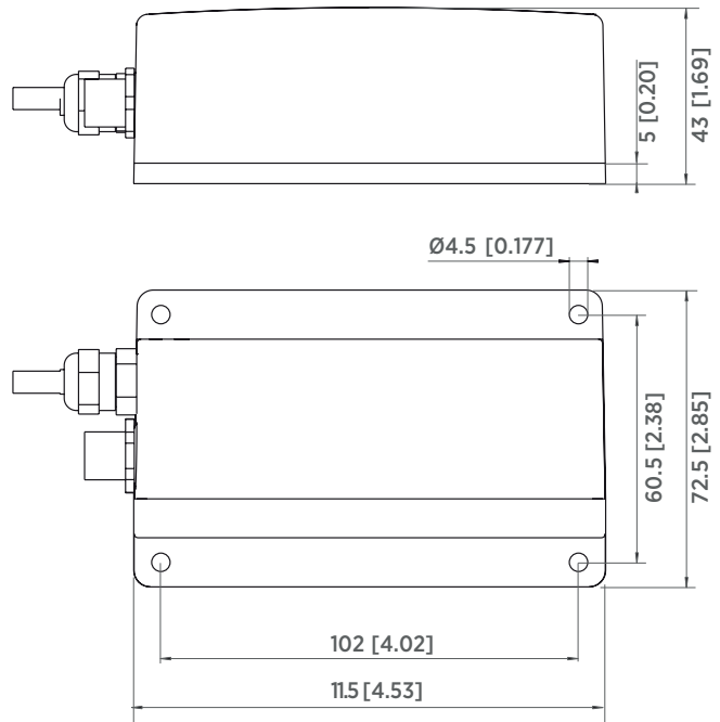
HMT310 Messwertgebergehäuse
