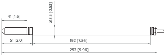
Sonde HMT315
