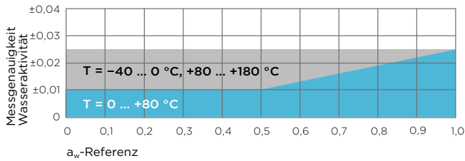
Messgenauigkeit Wasseraktivität
