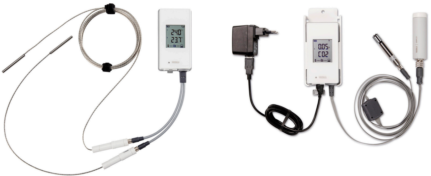
RFL100 mit zwei TMP115 Sonden (links) und mit GMP251 Sonde und HMP110 Sonde (rechts)
