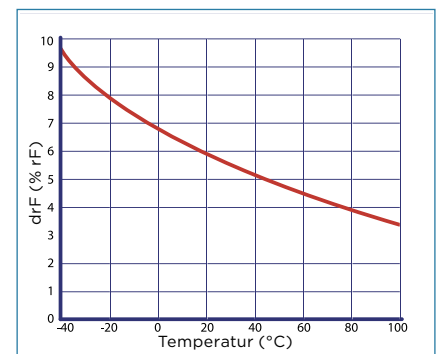
Abb. 2: Der Messfehler bei 100 % rF und verschiedenen Temperaturen, wenn der Temperaturunterschied zwischen Umgebungsluft und Sensor 1 °C beträgt.
