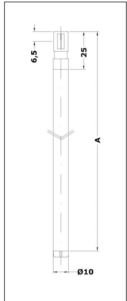
Sonde TA10 ... ZG1b (Maß A s. Seite 2)
